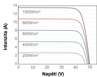
Křivka proudu a napětí JAM72S30-540/MR
