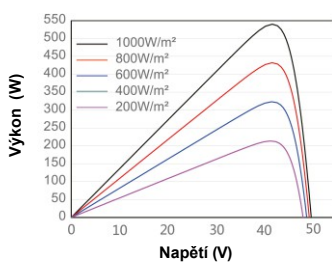
Křivka výkonu a napětí JAM72S30-540/MR
