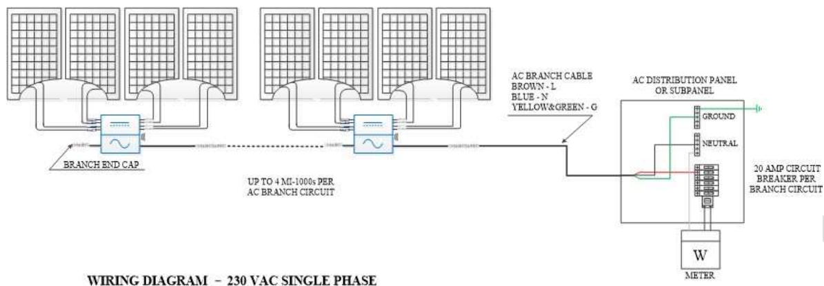
Rys. 2 Schemat połączeń jednofazowych
