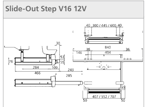
Slide-Out Step V16 12V Ducato
